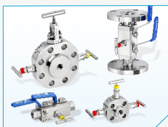
Двойные запорно-спускные краны (Манифольды 1 VM)
