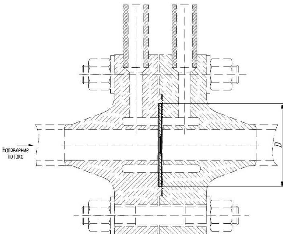
Рисунок 1.6 - Конструкция диафрагм типа ДВС с угловым способом отбора давления
